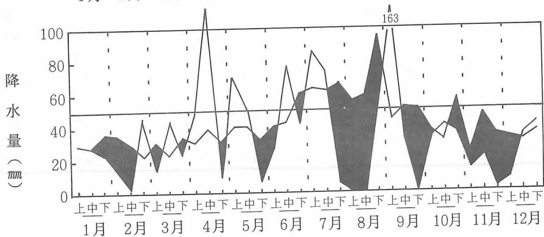
図 I-2 昭和59年の最高・最低気温と日照時間および降水量の推移(平年と比較)
