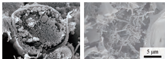
(写真左) クリプトスポリジウムのオシストの断面の電子顕微鏡像 (写真右) メタン発酵で活躍する微生物 Left: Intracellular structures of Cryptosporidium parvum oocyst. Right: Bacteria and archaea in the anaerobic digested reactor.
