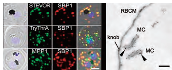
図1 質量解析で同定した各蛋白質(緑:STEVOR, TrypA, MPP1)とマウレル裂の構成蛋白質であるSBP1(赤)の共焦点顕微鏡解析による共局在の確認(原虫の核(青):左図)。MPP1(5nm金コロイド)とSBP1(15nm金コロイド)の赤血球膜(RBCM)近傍のマウレル裂(MC)内での相互作用(電子顕微鏡像:右図)。
