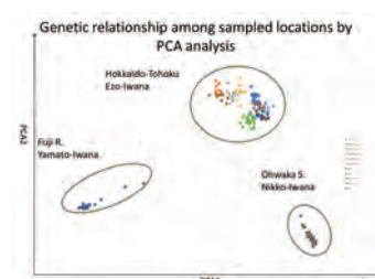
図2 イワナ地域集団の遺伝的差異 Fig. 2. Genetic population structure of Japanese charr.
