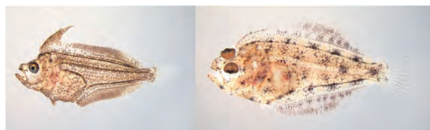
図3 ヒラメの変態:左右対称な仔魚から左右非対称な稚魚へ Fig. 3. Flatfish metamorphosis, transition from symmetric to asymmetric body plan.
