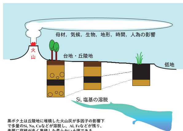
黒ボク土の生成過程模式図 Schematic diagram showing Andosol formation
