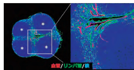
マウスのパイル板(腸管の二次リンパ組織)の濾胞(*)周囲に発達する血管とリンパ管 Blood vessel and lymph vessel around the follicular regions (*) of Peyer's patches in mice
