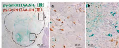
(左)ホタテガイの2種類のGnRHペプチド神経の分布
