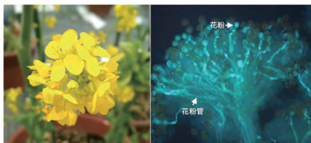
研究対象のアブラナ科の花と花粉管伸長の様子 Flowers of Brassica plants and the pollen tube elongation on stigma
