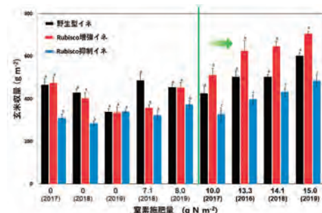
図2 2016年度から2019年度までの4年間のノヒカリ、Rubisco増強イネ、Rubisco抑制イネの玄米収量の結果。10 g N m -2 以上の窒素施肥区で、Rubisco増強イネの玄米収量が増加した(図中、矢印より右側)。
